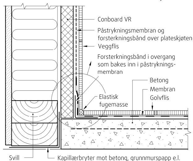
Fig. 3 Eksempel på overgang mellom fliskeledd golv og vegg med membran under flisene på golv.
