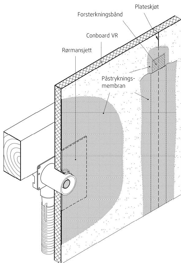
Fig. 2 Prinsipp for tetting rundt rørgjennomføringer og ved skjøter
