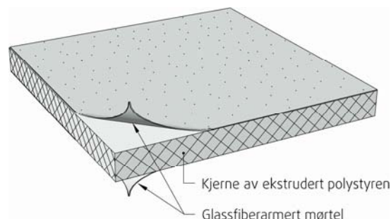
Fig. 1 Oppbygningen av Conboard VR. Platene er symmetriske med armert mørtel på begge sider
