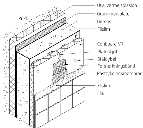
Fig. 4 Eksempel på bruk av Conboard VR på vegg under terreng.
